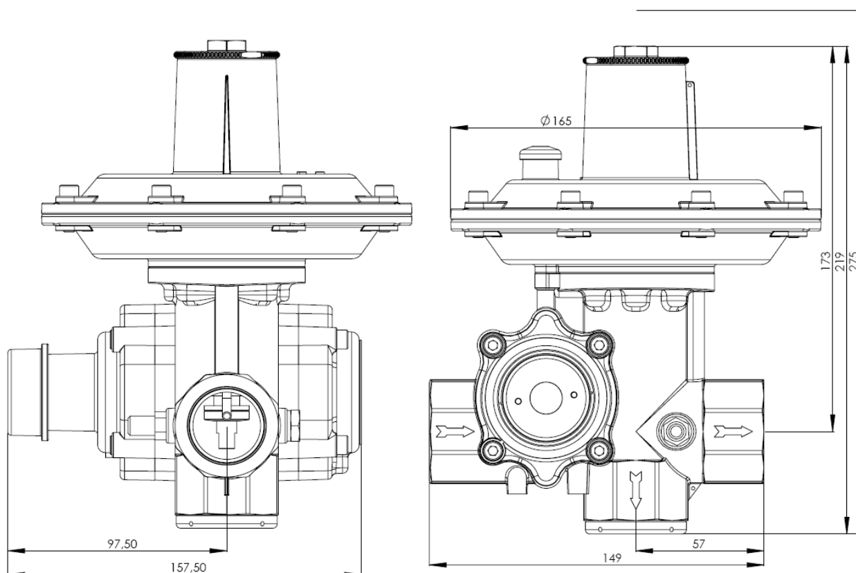
Figura 6 – Dimensiuni constructive ale RTG 25 cu supapă de blocare
