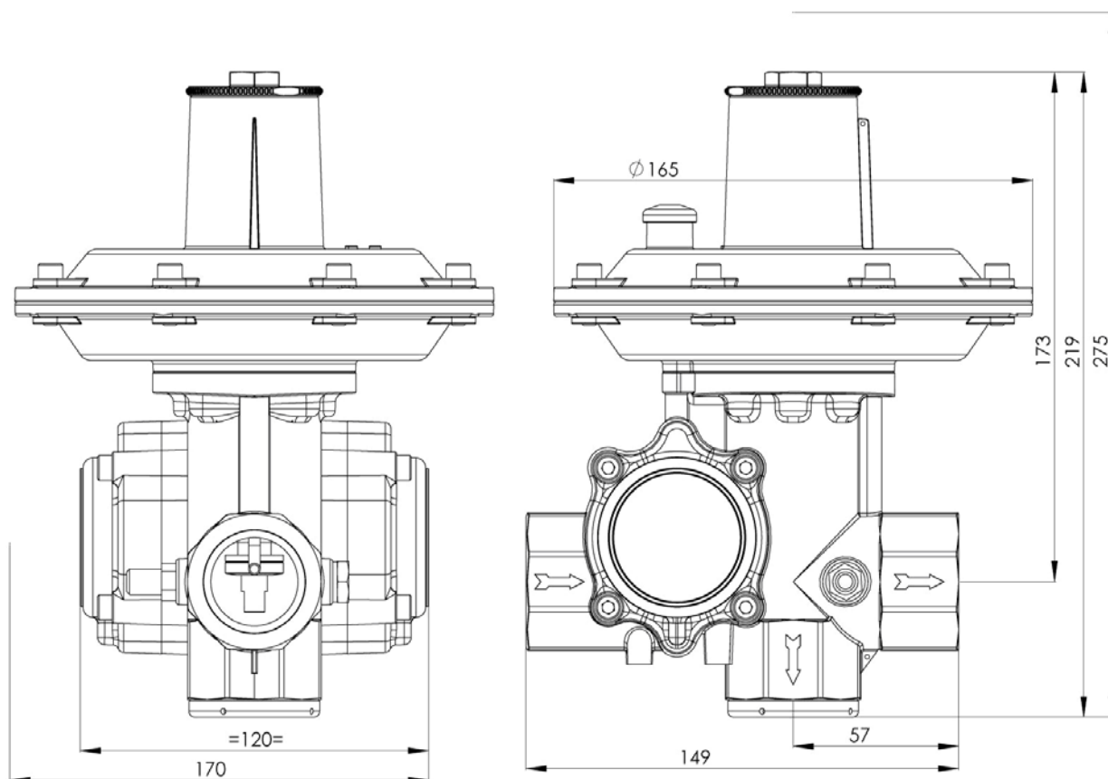
Figura 5 – Dimensiuni constructive ale RTG 25 fără supapă de blocare
