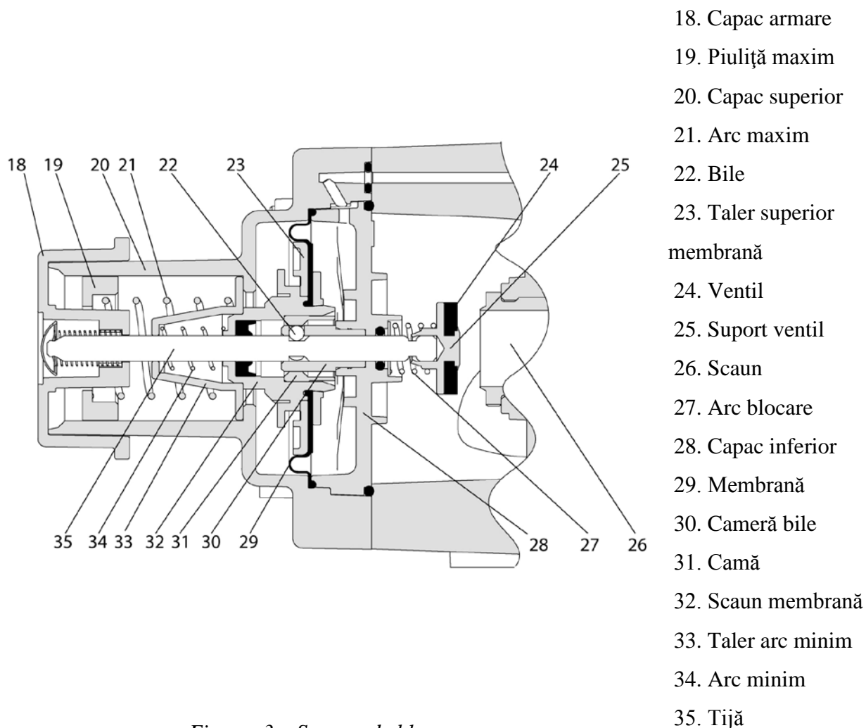
Figura 3 – Supapa de blocare
