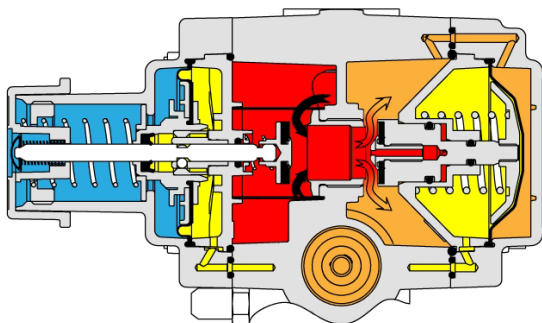
Figura 3 – regulator stadiul 1
