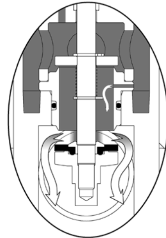
Figura 4 - Detaliu RTG 25 DB cu armare automată
